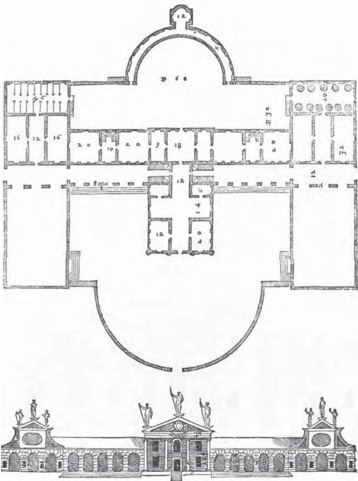
de los Quattro libri dell'architettura di Andrea Palladio, Venecia 1570
