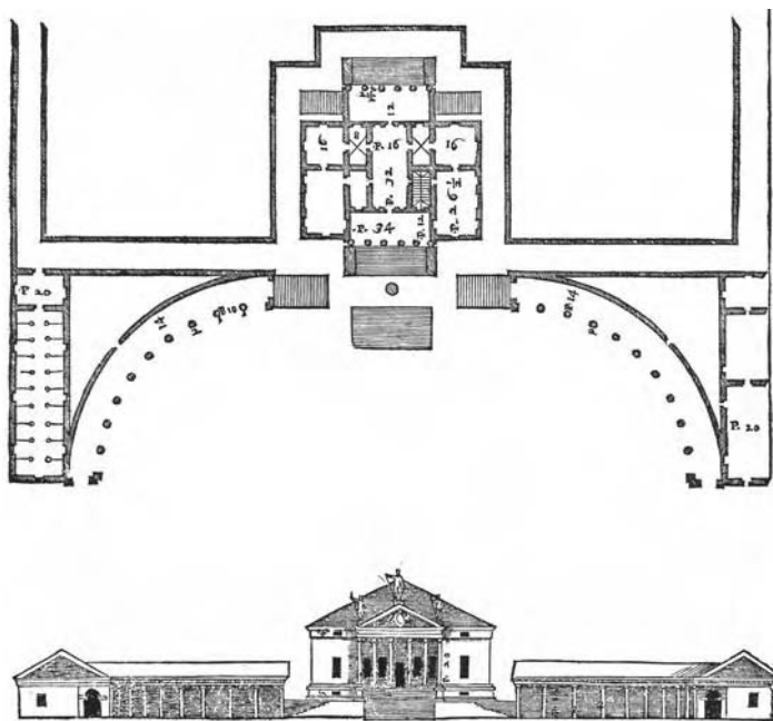
de los Quattro libri dell'architettura di Andrea Palladio, Venecia 1570
