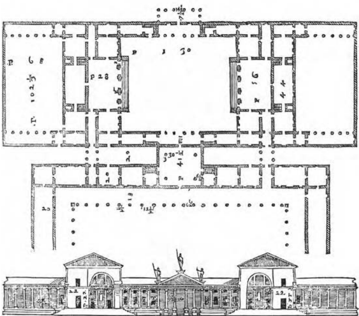
de los Quattro libri dell'architettura di Andrea Palladio, Venecia 1570
