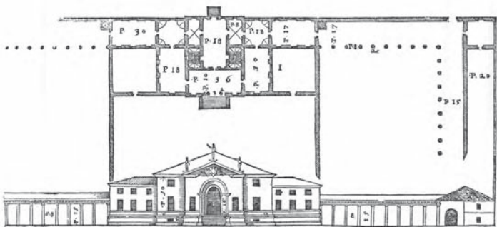
de los Quattro libri dell'architettura di Andrea Palladio, Venecia 1570
