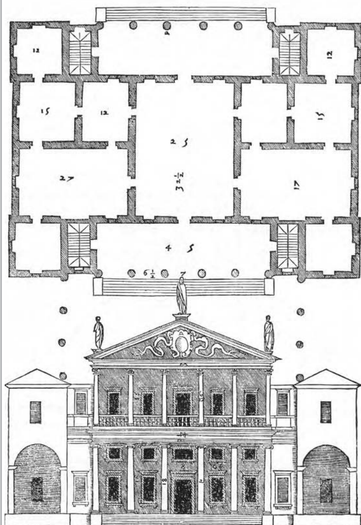
de los Quattro libri dell'architettura di Andrea Palladio, Venecia 1570
