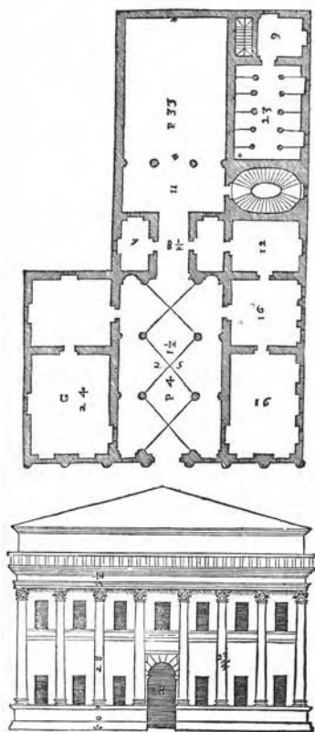
de los Quattro libri dell'architettura di Andrea Palladio, Venecia 1570
